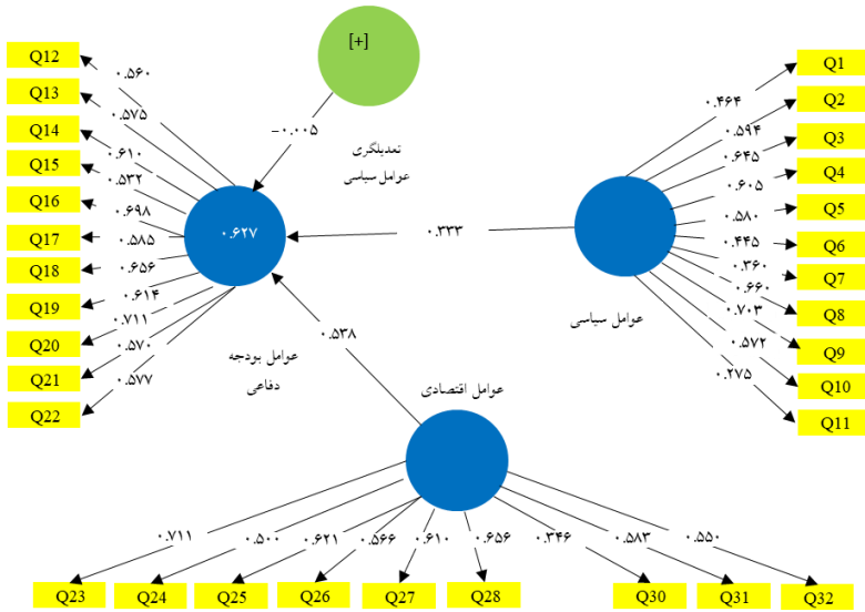
شکل شماره (۲) روابط بین مولفه‌ها و شاخص‌ها
