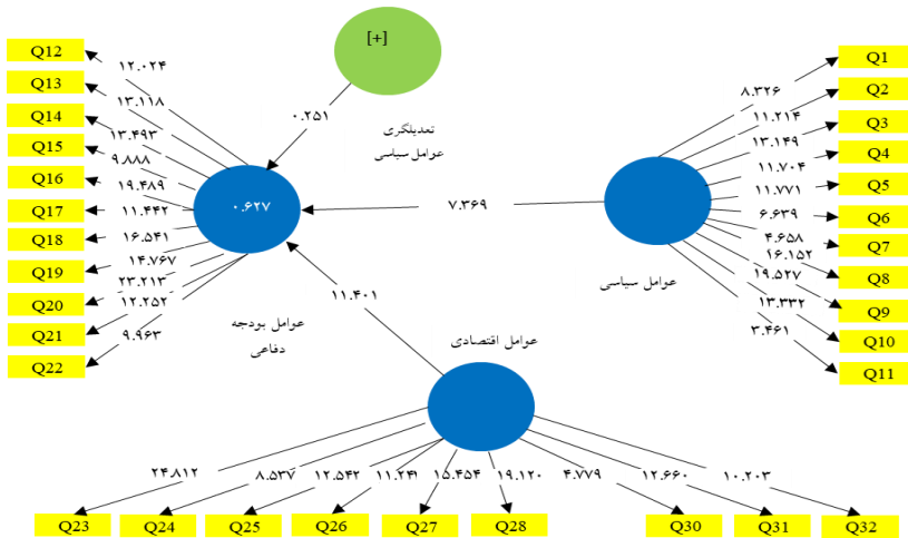
شکل شماره (۳) مقادیر T روابط بین متغیرها در مدل نهایی
